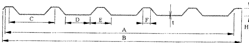
Obr. 1: Střešní a stěnový profil SAT35 Al
